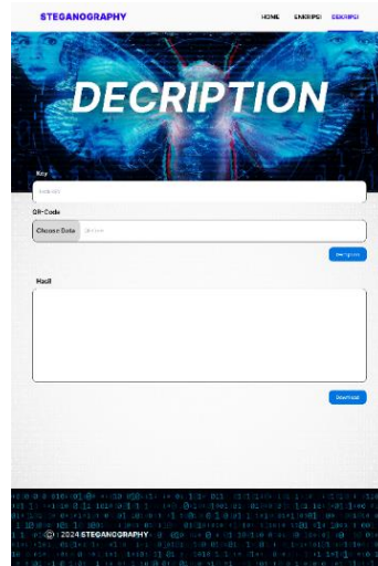
Gambar 9. Tampilan dekripsi
